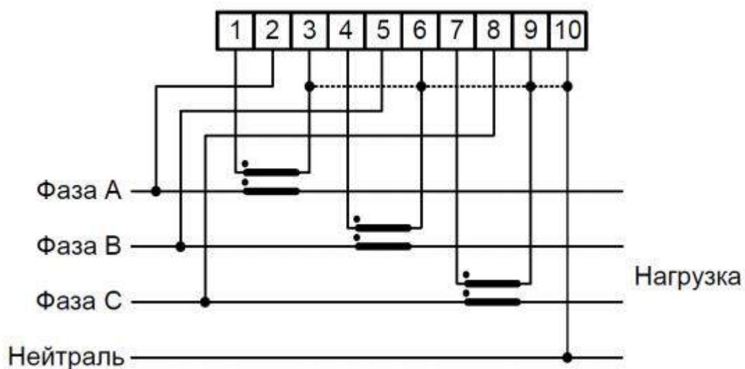
Рисунок 4. Схема подключения счетчика CE318 полукосвенного включения. Подключение через три трансформатора тока, трехфазная четырехпроводная сеть
