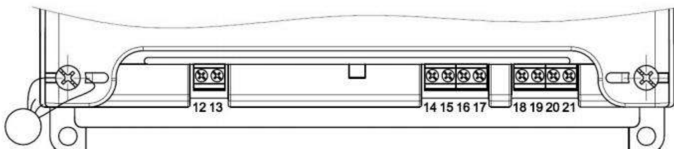
Рисунок 6. Обозначение функциональных контактов счетчика CE318 R32
