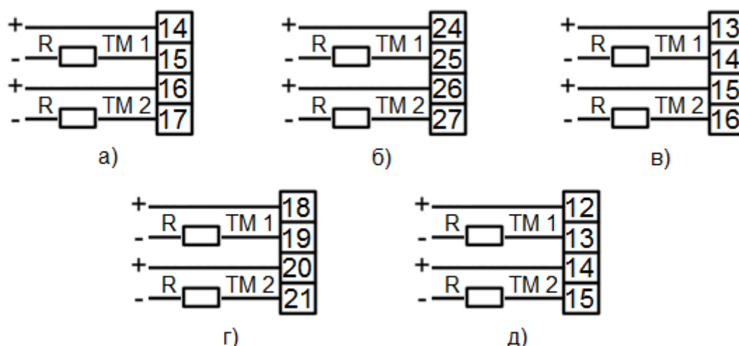
Рисунок 15. Схема подключения импульсного выхода
