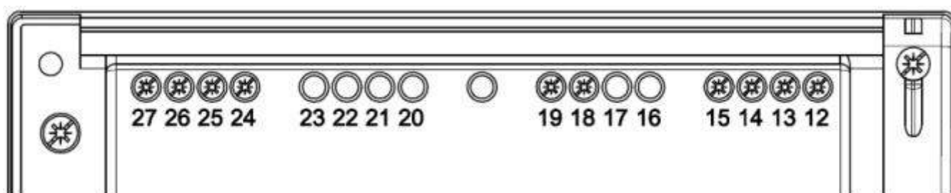
Рисунок 7. Обозначение функциональных контактов счетчика CE318 R33
