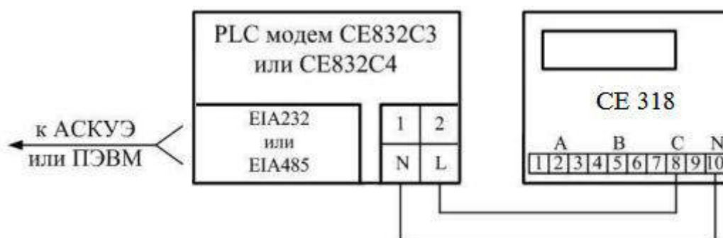
Рисунок 22. Схема подключения счетчика трансформаторного включения через PLC-интерфейс
