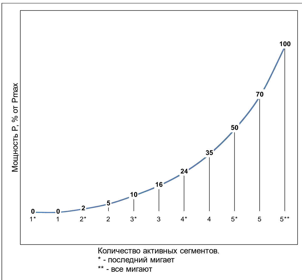
Рисунок 43. Зависимость индикатора активной мощности от фактического уровня активной мощности
