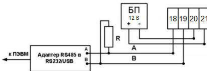
Рисунок 17. Схема подключения интерфейса RS-485 счетчика CE318 R32
