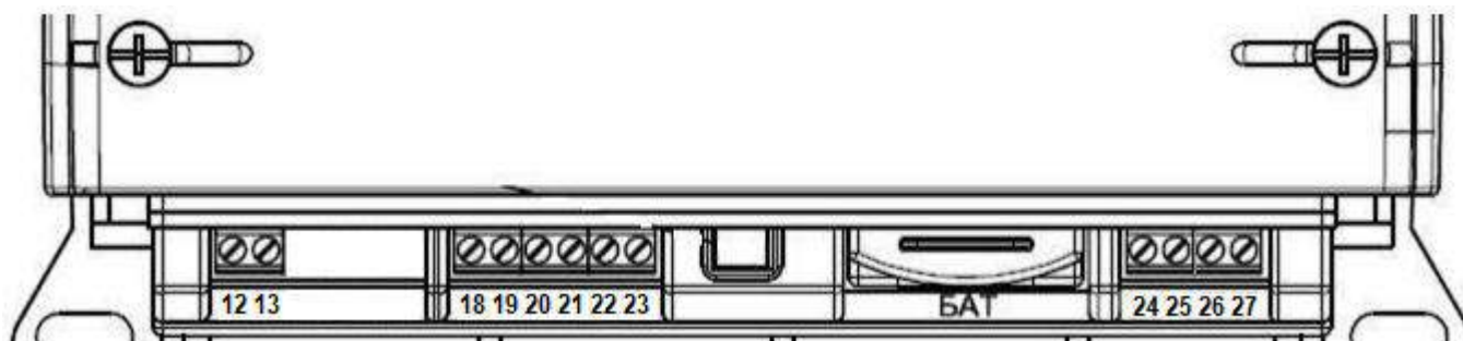
Рисунок 9. Обозначение функциональных контактов счетчика CE318 S35 xx3
