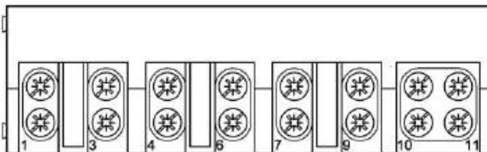
Рисунок 13. Обозначение контактов зажимов счетчика CE318 R3x (S3x) 746 (747)
