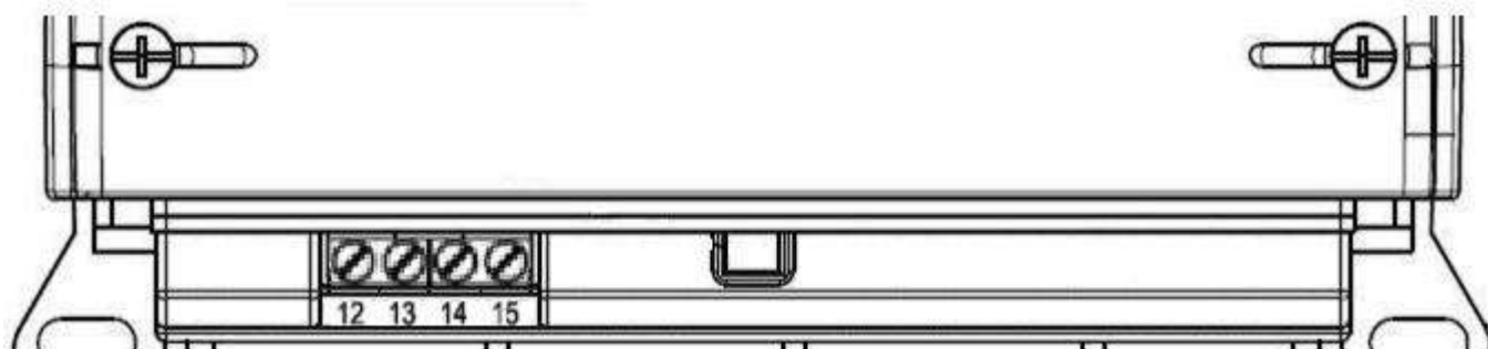
Рисунок 10. Обозначение функциональных контактов счетчика CE318 S35 74x (14x, 84x)
