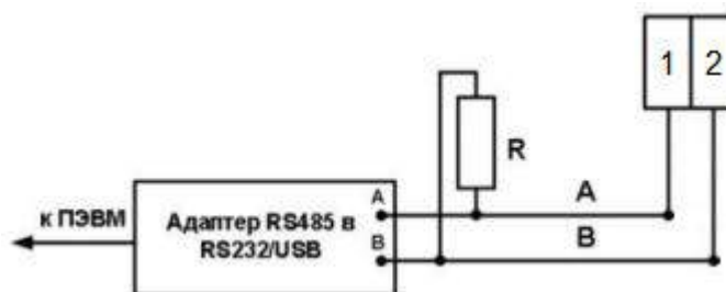
Рисунок 19. Схема подключения интерфейса RS-485 счетчика CE318 S31 (S34)
