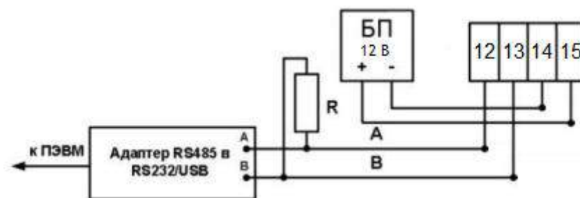
Рисунок 18. Схема подключения интерфейса RS-485 счетчика CE318 R33
