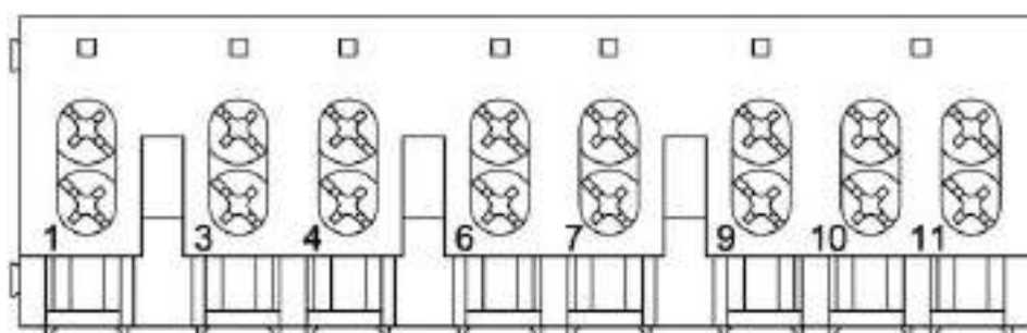
Рисунок 12. Обозначение контактов зажимов счетчика CE318 R3x (S3x) 745 (749)
