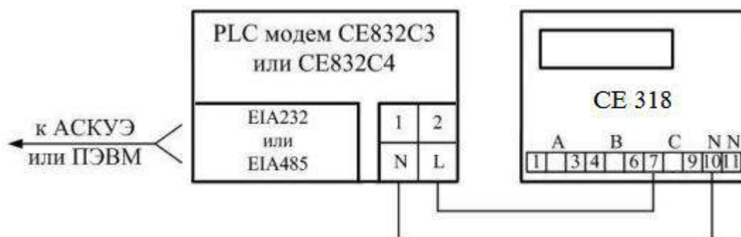
Рисунок 23. Схема подключения счетчика прямого включения через PLC-интерфейс
