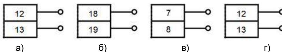
Рисунок 16. Схема подключения реле сигнализации
