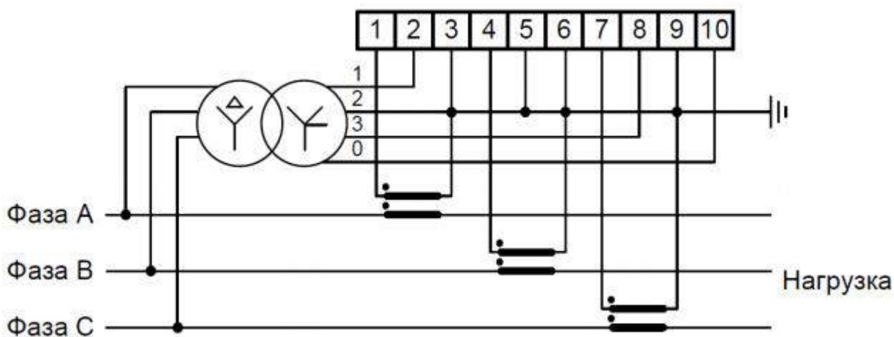
Рисунок 5. Схема подключения счетчика CE318 трансформаторного включения. Подключение через три трансформатора тока и три трансформатора напряжения, трехфазная трехпроводная сеть.
